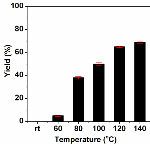
Hình 5 Ảnh hưởng của nhiệt độ đến độ chuyển hóa phản ứng
