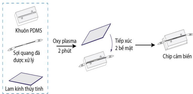
Hình 2 Quy trình chế tạo kênh dẫn vi lỏng cho cảm biến quang học.
