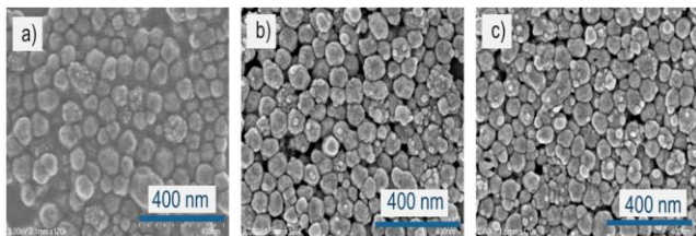
Hình 6 Ảnh SEM của lớp phủ \text{Ag@Au} NPs trên nền \text{SiO}_2 theo thời gian (4, 6, 8) giờ.
