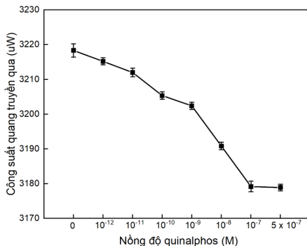
Hình 7 Sự phụ thuộc của công suất quang đầu ra theo nồng độ quinalphos trên nền vật liệu \text{Ag@Au} NPs.
