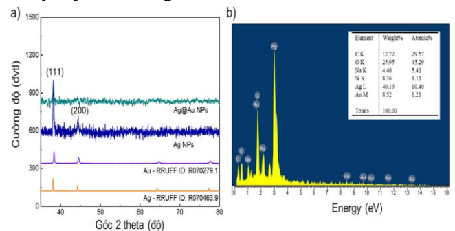
Hình 5 a) Biểu đồ nhiễu xạ tia X của mẫu Ag NPs và Ag@Au NPs; b) Phổ EDX của mẫu Ag@Au.
