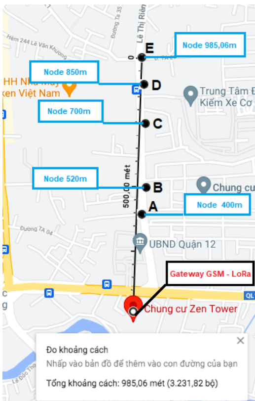
Hình 11 Đo khoảng cách truyền trong đô thị
