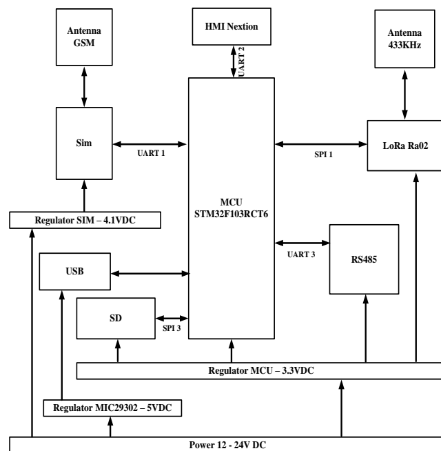
Hình 5 Sơ đồ khối cổng chuyển đổi
