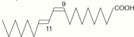
9 c ,11 t -18:2
