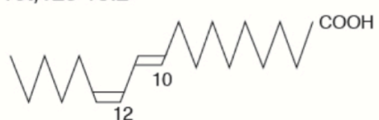
10 t ,12 c -18:2
