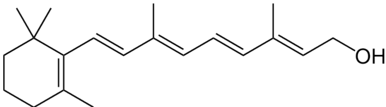
Retinol
